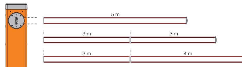
M7BAR Con asta da 5 m Predisposta per: gomma protettiva, luci di segnalazione, rastrelliera (2 pz), appoggio mobile
