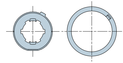
515.25001 Tondo con nervature e con linguetta interno 47 ruota + corona ad anello
