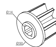
575.12150 Calotta senza perno per rullo Ø 50 mm.
