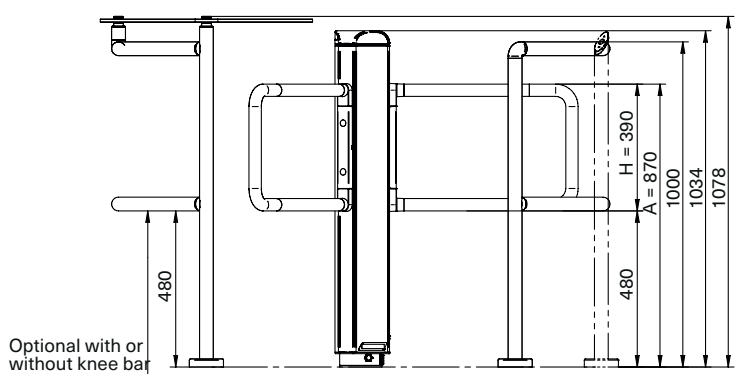
mTwing con barre a U - vista laterale
