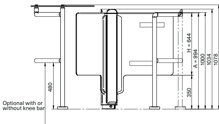
mTwing con pannelli in vetro - vista laterale
