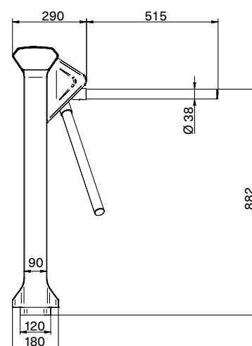
mTripod corto – vista frontale
