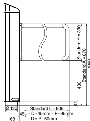
mSwing con barra a U – vista frontale
