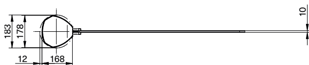
mSwing – vista dall'alto
