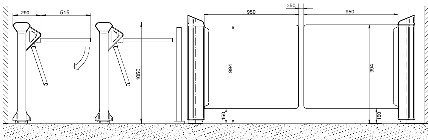
Configurazione di linea con mTripod e mSwing come varco a doppio battente
