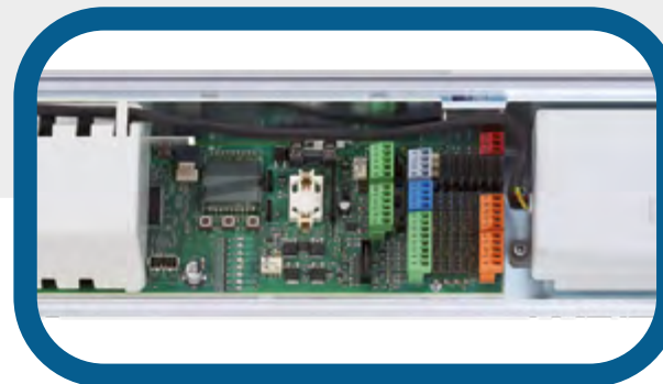
Unità di controllo E1SL con alimentatore "switching" a basso consumo (stand-by &lt;3W)
