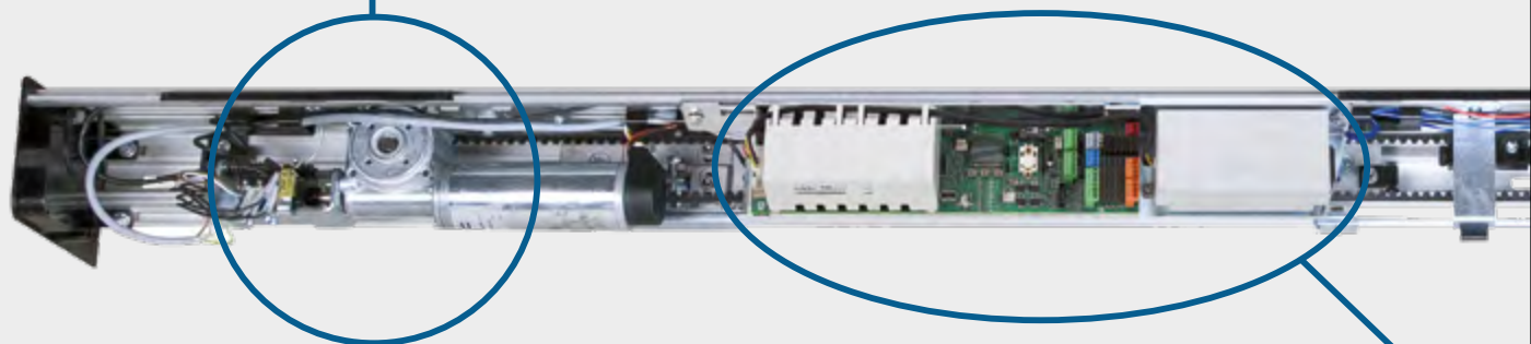
Unità di controllo E1SL con alimentatore "switching" a basso consumo (stand-by &lt;3W)
