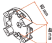
TM2 45 supporto standard in plastica (6 fori per viti M5) MAX 15Nm
