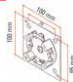
TM2 45 supporto plastico universale con base in acciaio 100x100mm MAX 15Nm
