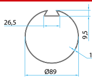
TM2 45 adattatore per tubo Deprat 89
