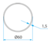
TM2 45 adattatore per tubo tondo 60mm
