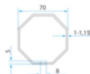
TM2 45 adattatore per tubo ottagonale 70mm
