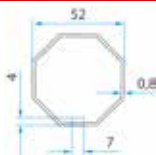
TM2 45 adattatore per tubo ottagonale 52mm
