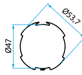
TM2 45 adattatore per tubo ZF 54mm
