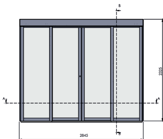
SKR35 SEZIONI
